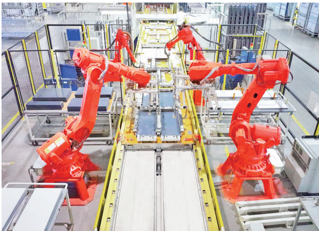
▲海尔重庆冰箱互联工厂内的门面压合全自动线
